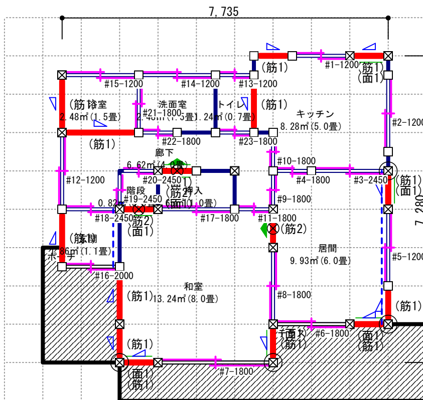
1階
