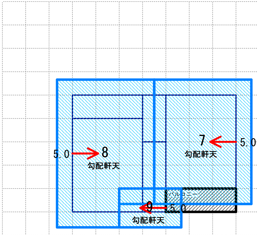
2階
