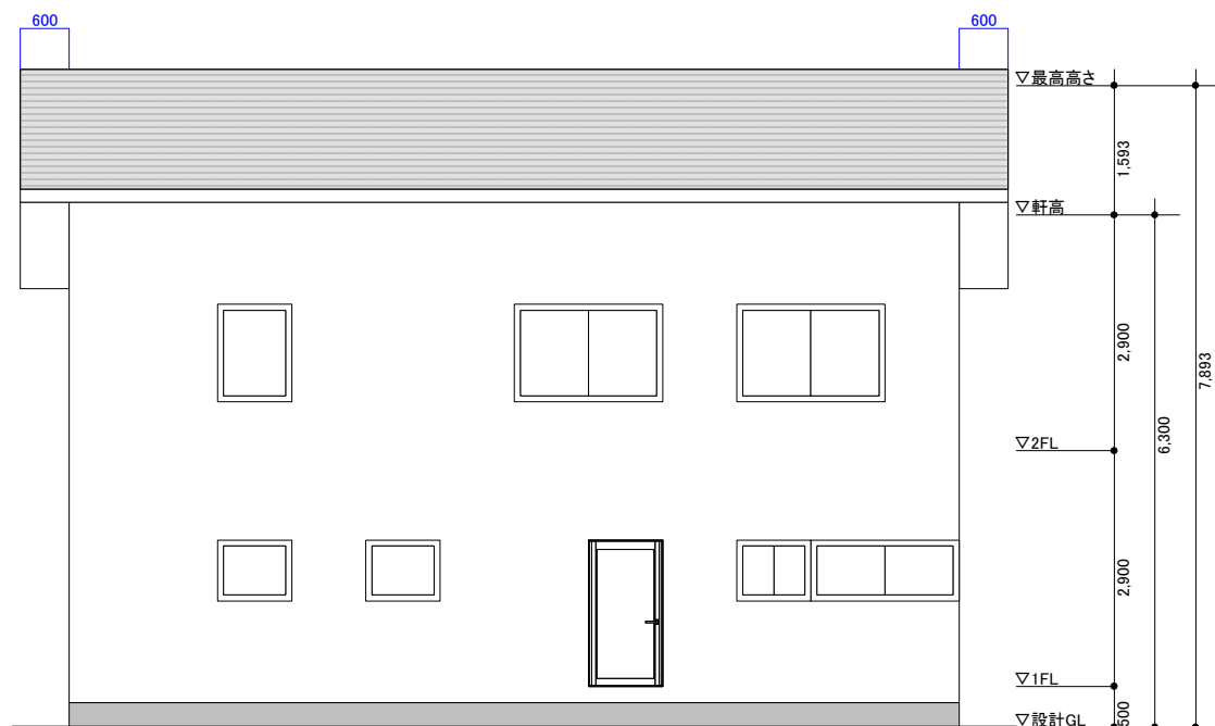
北立面図
