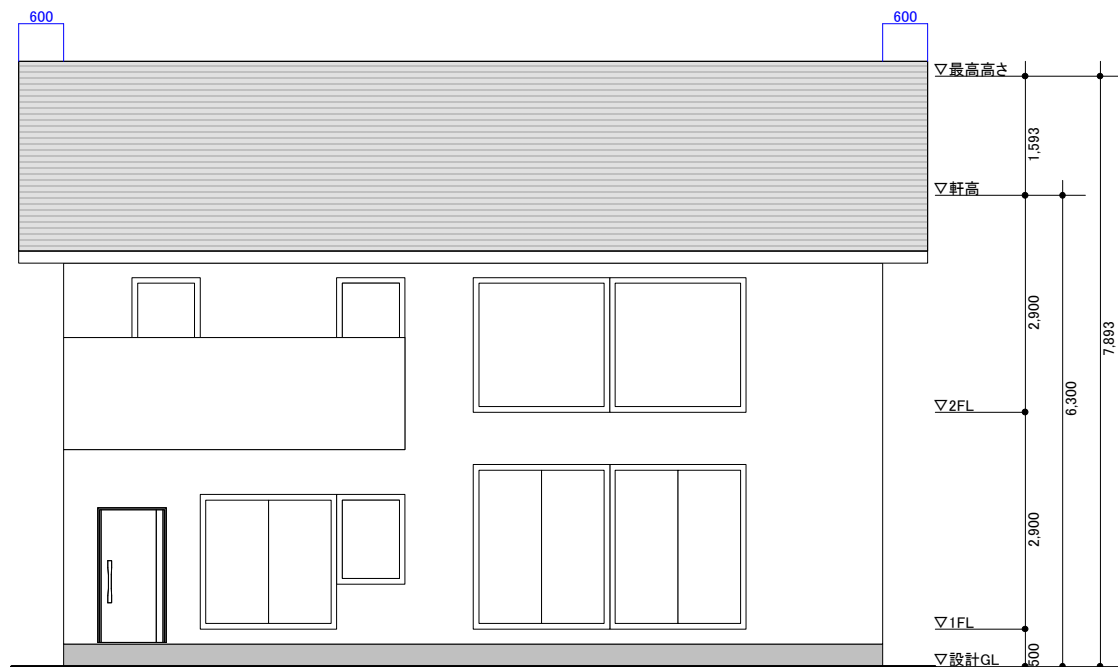
南立面図
